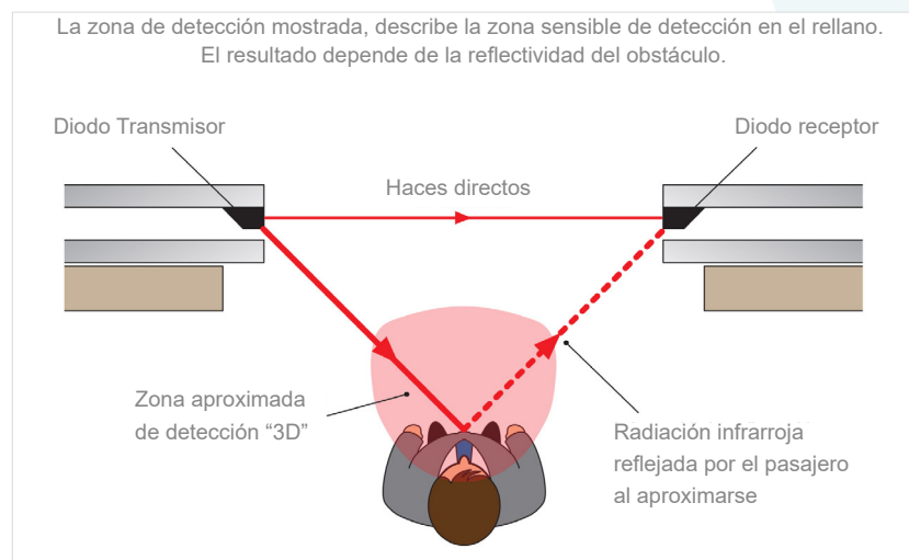
Fig 3: Esquema de funcionamiento del sistema Pana40+3D mostrando la zona sensible de detección en el rellano
